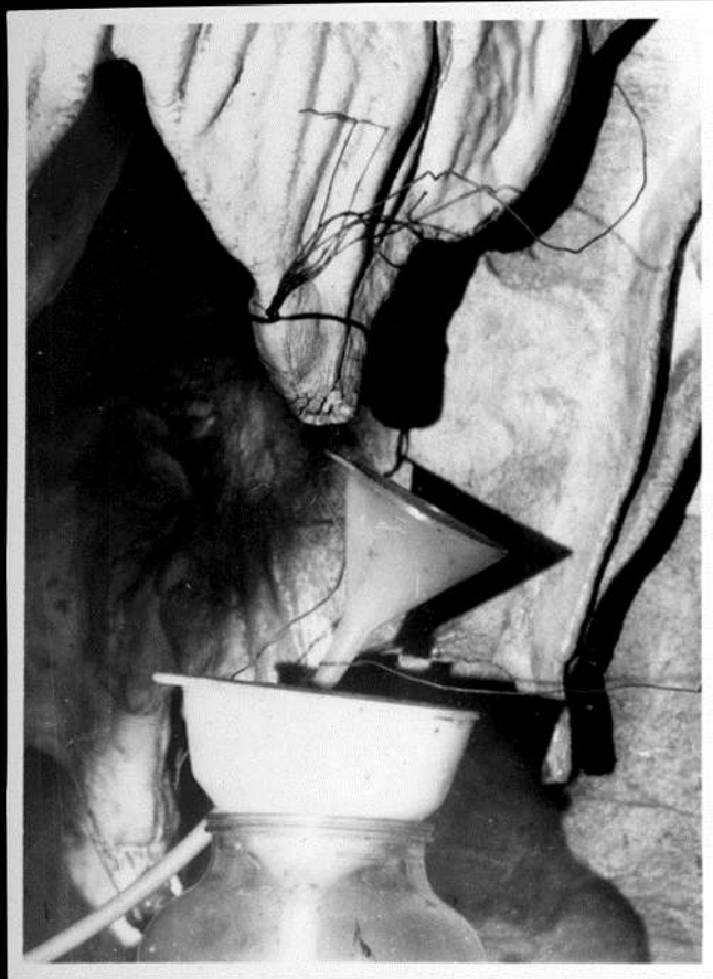
A 7-ES CSEPEGÉSMÉRŐHELY A LÉTRÁSI-VIZES-BARLANGBAN
