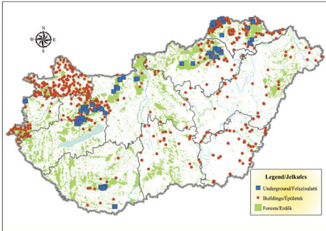
3. ábra. A végrehatása során adatgyűjtéssel érintett felszínalatti objektumok és épületek.
