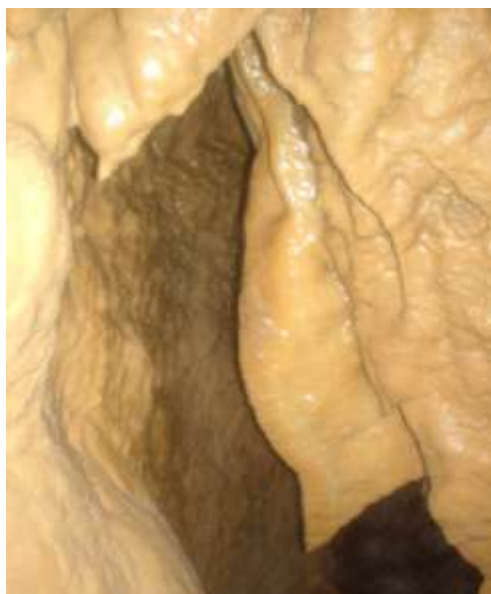
6. ábra: Cseppkőzászló
