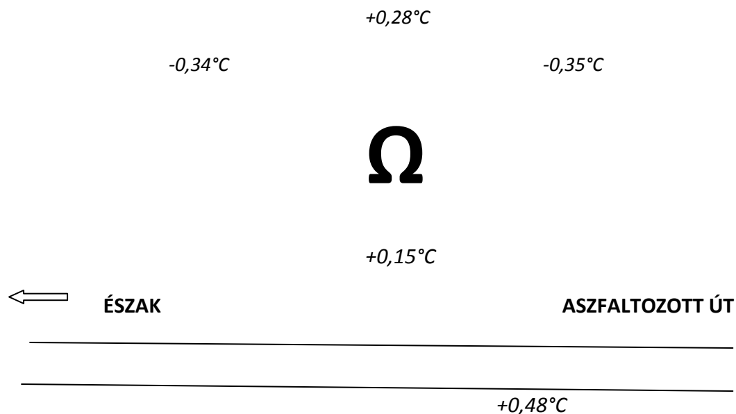
7. sz. ábra: a talajhőmérsékletek tipikus eloszlása barna erdei talaj esetében, 10 cm mélységben. A mérés 2015 januárban történt, amikor a levegő hőmérséklete -1,8°C volt. A tapasztaltak megegyeznek az 1 évvel korábban rögzítettekkel.
