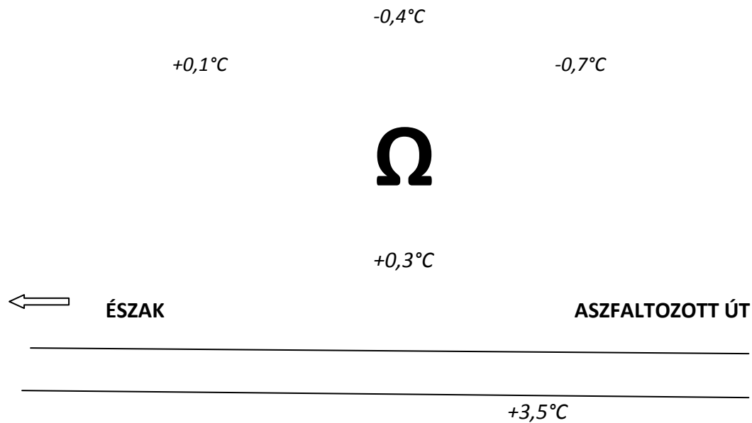
7. sz. ábra: a talajhőmérsékletek tipikus eloszlása barna erdei talaj esetében, 10 cm mélységben. A mérés 2014 januárban történt, amikor a levegő hőmérséklete 9,8°C volt, azonban az elmúlt hetekben rendszeres éjszakai fagyok voltak. Látható, hogy az aszfaltozott út fölött 10 méterre nyíló barlangbejárat körül - a hegyoldalról lecsorgó hideg levegő hatására – a talaj átfagy, míg az aszfaltozott út túloldalán (10 méterre a barlang bejáratától) már enyhébb hőmérsékleti viszonyok tapasztalhatók. A talajhőmérséklet 10 cm méter mélységben a hónapos átlag csúsztatott, integrált értékét mutatja
