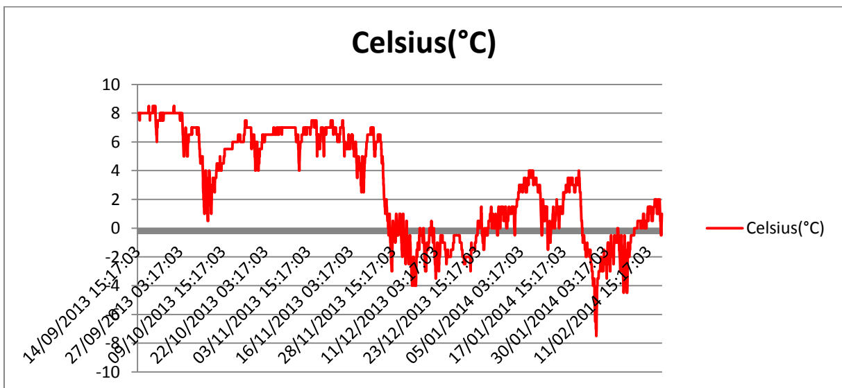
3. sz. diagram: a barlangi hőmérséklet menete 2013 őszétől 2014 februárig terjedő időszakban. Látható, hogy decembertől februárig a barlangba befelé áramlik a hideg felszíni levegő, mely lehűti a járatokat és ott jeget rak le. A lehűlés mértéke sokkal kisebb, mert 2013 tele sokkal enyhébb volt, mint a 2012-es. A jég mennyisége is kevesebb volt a barlangban.
