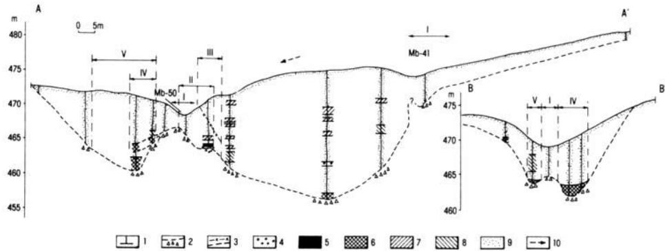
9. ábra. A Mester-Hajagon az Mb-50 jelű karsztos mélyedés környékének üledékföldtani szelvényei (VERESS M.—FUTÓ J.—HÁMOS G. 1986, módosítva). - 1 = fúrás hely; 2 = fúrással elért mészkőfelek; 3 = feltételezett hajdani és jelenlegi mészkőfelek; 4 = kavics; 5 = barna agyag; 6 = vörösbarna agyag; 7 = laminit; 8 = eltemetett talaj; 9 = lösz, agyagos lösz; 10 = hajdani anyagszállítás, I. rejtett kőzethatáron kialakult recens mélyedések (Mb-50: karsztosodással szétromcsolt kiemelkedés tetején, Mb-41: kiemelkedés oldalában), II. karsztosodással lepusztult kiemelkedés (a vörösbarna agyag hiánya jelzi, hogy környezete fölé magasodó lepusztulási térszín volt), III. a kúp hajdani karsztosodó oldala (a felületét metsző laminitösszletek tavak szintjeit, tehát a kőzethatár eltolódását jelzik), IV. a kúp lejtőjén és mélyedéseibe áthalmozódva megnövekedett vastagságú vörösbarna agyag, V. feltehetően fosszilis mélyedés (kialakulását követően vörösbarna agyag, lösz, majd nagy vastagságban talaj töltötte ki)
