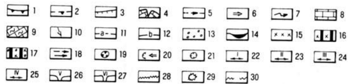
5. ábra. Karsztosodás, a völgytengellyel megegyező irányú és a völgy alá eső eltemetett kúpokon (a Hidegaszó-völgy példáján). - 1 = laza üledékben képződött völgyoldal; 2 = laza üledékben képződött hajdani völgyoldal; 3 = mészkőben képződött völgyoldal; 4 = antiklinális völgy oldalnézetben; 5 = időszakos vízfolyás; 6 = vízáramlás a felszínen és vízzáró felett; 7 = vízelszivárgás; 8 = felsőjúra mészkő; 9 = középsőkreta mészkő; 10 = feltételezett vető; 11 = kavicsstakaró hajdani szintjei (a 1 ; a 2 ; a 3 ); 12 = jelenlegi felszín; 13 = kavics; 14 = agyag; 15 = löszös üledék; 16 = agyagos üledék; 17 = áthalmozott kevert kavics, agyag, iszap; 18 = fedőüledékek hajdani és jelenlegi áthalmozódása; 19 = inaktív víznyelőbarlang felülnézetben; 20 = víznyelő töbrök felülnézetben; 21 = utánrogyásos töbrök; 22 = teljesen elpusztult víznyelők zónája; 23 = inaktív víznyelők, víznyelő töbrök zónája; 24 = víznyelő töbrök zónája; 25 = utánrogyásos töbrök zónája; 26 = inaktív víznyelőbarlang oldalnézetben; 27 = aktív víznyelő töbrök oldalnézetben; 28 = kőzethatár; 29 = rejtett kőzethatár; 30 = nem aktív kőzethatár; A = felülnézet, B = oldalnézet
