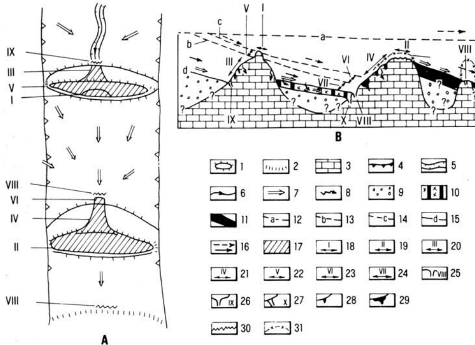
6. ábra. Karsztosodás a völgytengelyre merőlegesen elhelyezkedő, exhumálódó mészkőháton (a K-1 jelű víznyelő völgyének, valamint a Klein-pusztai-völgy példáján). - 1 = mészkőhát; 2 = mészkőhát tetősíntjének határa; 3 = mészkő; 4 = völgyoldal; 5 = víznyelő medre; 6 = vízfolyás; 7 = vízáramlás a felszínen és vízzáró felett; 8 = vízelszivárgás; 9 = kavics; 10 = agyagos üledék; 11 = agyagos mállástermék; 12 = hajdani kavicsstakaró; 13 = a lösz felhalmozódása előtti völgytalp; 14 = hajdani löszelborítás; 15 = a jelenlegi felszín; 16 = fedőüledék hajdani és jelenlegi áthalmozódása; 17 = karsztosodott zóna felülnézetben; 18 = oldásos töbrök zónája; 19 = utánrogyásos töbrök zónája; 20 = inaktív víznyelők sávja; 21 = inaktív víznyelők és utánrogyásos töbrök sávja; 22 = inaktív víznyelő töbrök és utánrogyásos töbrök zónája; 23 = inaktív víznyelő töbrök (hajdani víznyelők) sávja; 24 = inaktív víznyelő töbrök sávja; 25 = aktív víznyelő töbrök; 26 = aktív víznyelő; 27 = rejtett víznyelőképződés; 28 = eltömődött vízelvezető járat oldalnézetben; 29 = fosszilis (feltöltődött) karsztos mélyedés oldalnézetben; 30 = jelenlegi kőzethatár; 31 = a karsztos mészkő hajdani felszíne; A = felülnézet, B = oldalnézet
