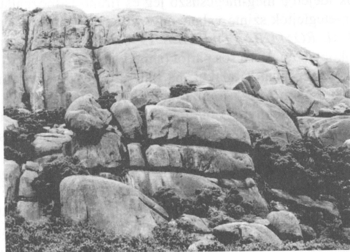
2. kép: Gyapjúzsákok az O Pindo-hegységből Picture 2.: Woolsacks in the O Pindo Mountains
