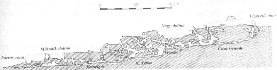
4. ábra: Az O Folón-barlangrendszer metszete (Felmérte a Maíxo Barlangkutató Klub 1990-2007 között) Fig. 4.: Profile of the O Folón Cave System (Surveyed by Maíxo Speleologic Club between 1990-2007)
