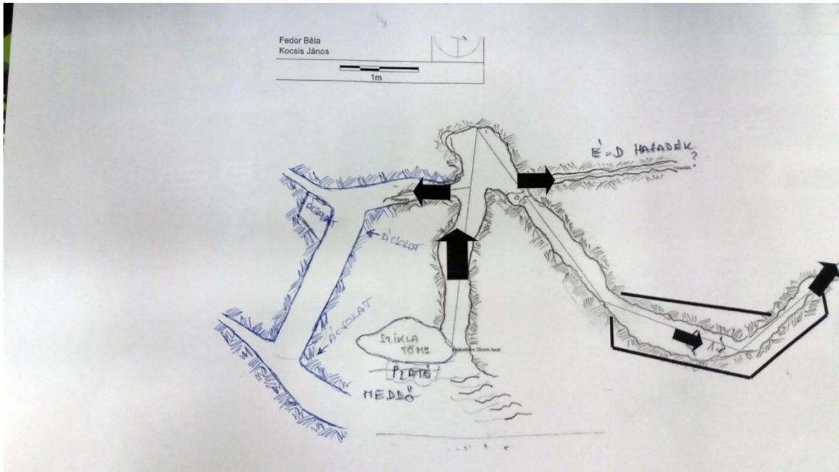
4. sz. ábra: a barlang felméréséről készült korábbi munkatérkép (vízszintes szelvény), melyen jól látszik a több részletben kibontott, 70°os lejtésű kisakna és annak ellaposodó, feltöltött folytatása, mely a műút irányába fordul. (rajzolta: Kocsis János kutatásvezető-helyettes)
