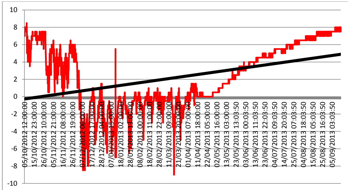
1. sz. diagram: a barlangi hőmérséklet menete 2012 őszétől 2013 őszéig terjedő időszakban. Látható, hogy decembertől áprilisig a barlangba befelé áramlik a hideg felszíni levegő, mely lehűti a járatokat és ott jeget rak le. Áprilistól szeptemberig megfordul a légáramlat, és a lehűlt barlangi levegő folyamatosan visszamelegedve áramlik a felszín felé.
