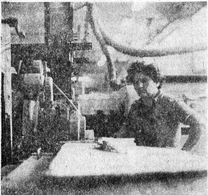
A Sátorlajújhelyi Dohánygyárban NDK-gyártósorokon készülnek a termékek. Felvételiünkön a jelenleg legmodernebb berendezés látható; a GARANT 20 MAX-cascade típusú filteres cigarettagyártó gép nyolc óra alatt 800 000 darab Symphoniát képes előállítani.
