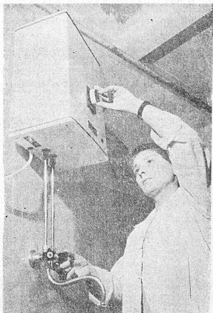
A Villamos Berendezés és Készülék Művek gyártmány-fejlesztési intézetének legújabb készítménye a hőfokszabályozóval, keverőcsatléppel ellátott 10 literes melegvíz-tároló. Az új készítmény sorozatgyártására a harmadik negyedévében kerül sor.
