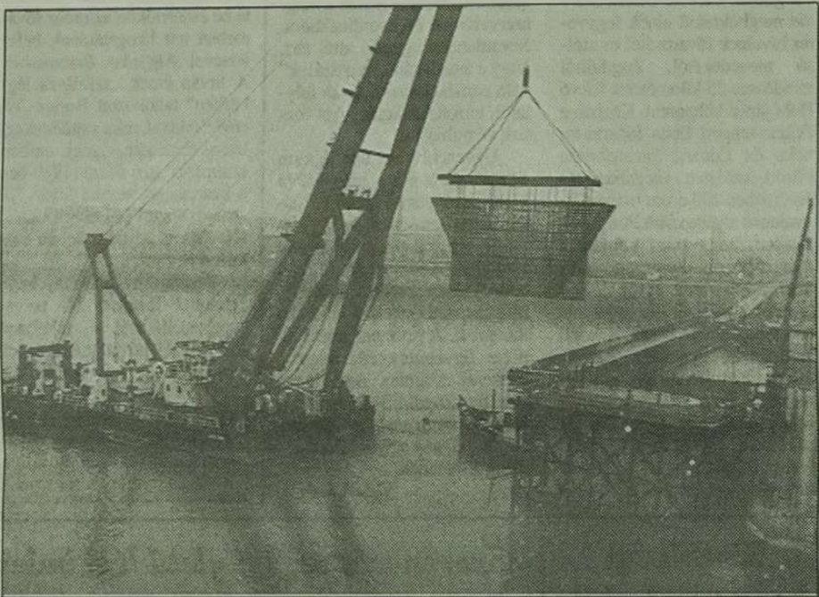
A Hídépítő Rt. tegnap a lágymányosi új Duna-híd építésénél beemelte a második mederpillér vasszerkezeti elemét
