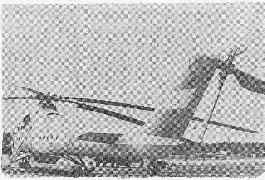
A szovjet repülőgépipar nagyszerű alkotásával, a MI-10 helikopterrel több világrekordot ért el. A legújabb csúcs: 25 105 kilogramm felemelése 2800 méter magasságra. Képünkön: a MI-10 helikopter.
