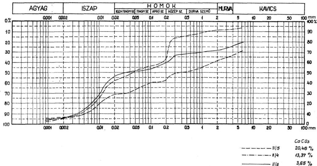
6. kép. A Diósgyőr—Tapolca barlang szemcseösszetételi görbéje
