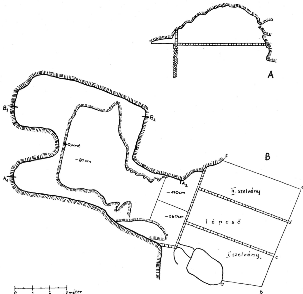
1. kép. Diósgyőr—Tapolca barlang: A) A barlang bejárata, B) A barlang és a szelvények alaprajza
