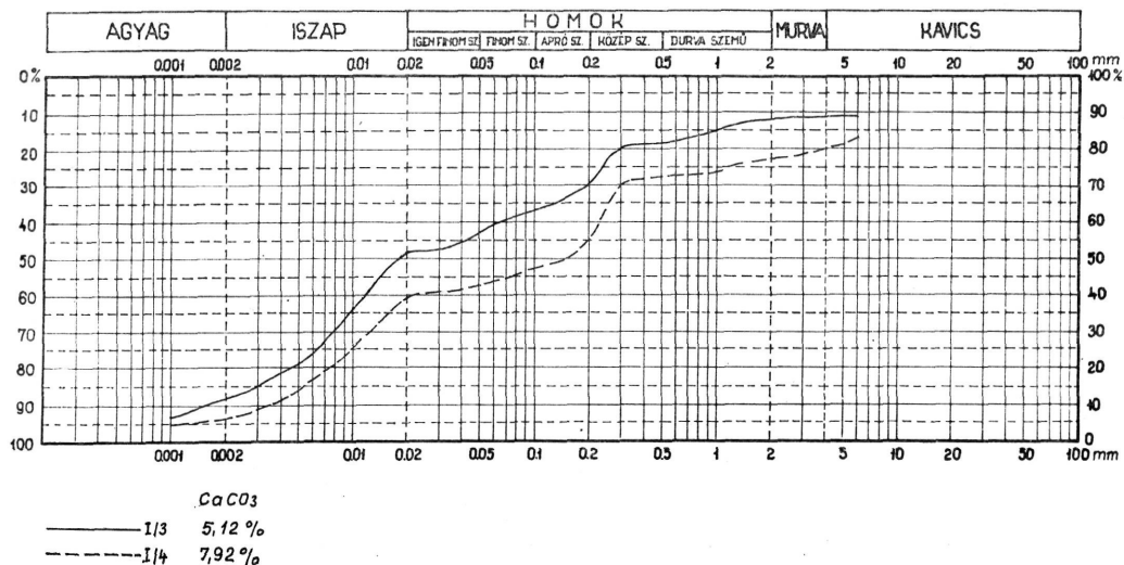
7. kép. A Diósgyőr—Tapolca barlang szemcseösszetételi görbéje
