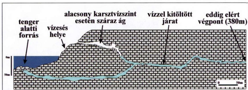
A Kotori-öbölben fakadó Sopot-forrás barlangjának hosszmetszete (Stefanovic et al. 2010 alapján)
