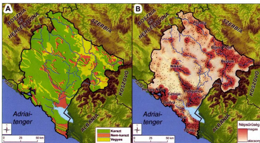
A) Karsztos, nem-karsztos és vegyes kőzetű területek Montegróban.
