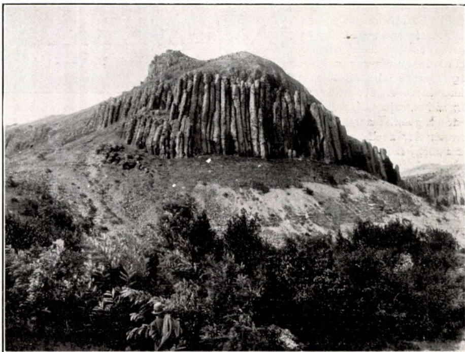
A Szent György-hegy bazaltoszlopai. Lóczy L. felvétele.
