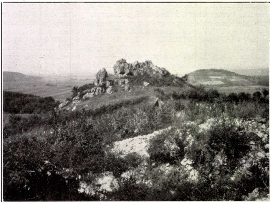
Tihany, Aranyház-gejzirkúp. Cholnoky J. felvétele.
