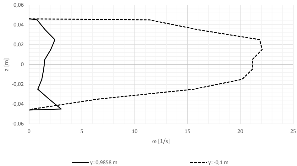
7. ábra: Örvényesség ( \omega ) értékeinek alakulása z tengely (mélység) irányában egy becsatlakozás előtt és után választott keresztmetszéken a 70^\circ -okkal becsatlakozó mellékvályút fogadó fővályúban, 5^\circ -os dőlésszög esetén. Fig. 7.: Tendency of vorticity ( \omega ) values along axis z (depth) in a selected cross section before and after the junction point of side and main channel with 70^\circ junction angle in case of 5^\circ slope angle.
