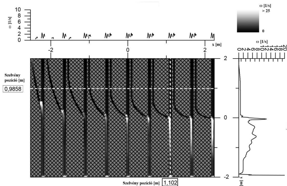
8. ábra: 5°-os dőlésszög esetén, 4 cm mélyen létrejövő örvényesség ( \omega ) a digitális vályúsorozat modellben. Az örvényesség ( \omega ) értékeinek változását hossz és kereszt-szelvény mentén részletesen lehet vizsgálni. Fig. 8: Vorticity ( \omega ) of the digital channel serial model in 4 cm depth in case of 5° slope angle. Change of vorticity ( \omega ) data is examinable in detail along cross and length sections.
