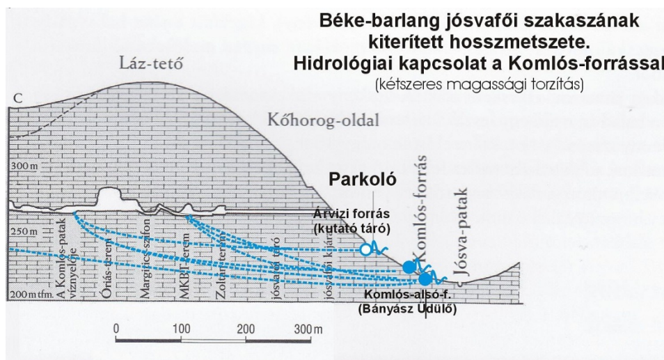
21. ábra A Béke-barlang jósvafői szakaszának hosszmetsete a lehetséges vízáramlásokkal (KISBÁN - SZUNYOG 2004. alapján, kiegészítve)
