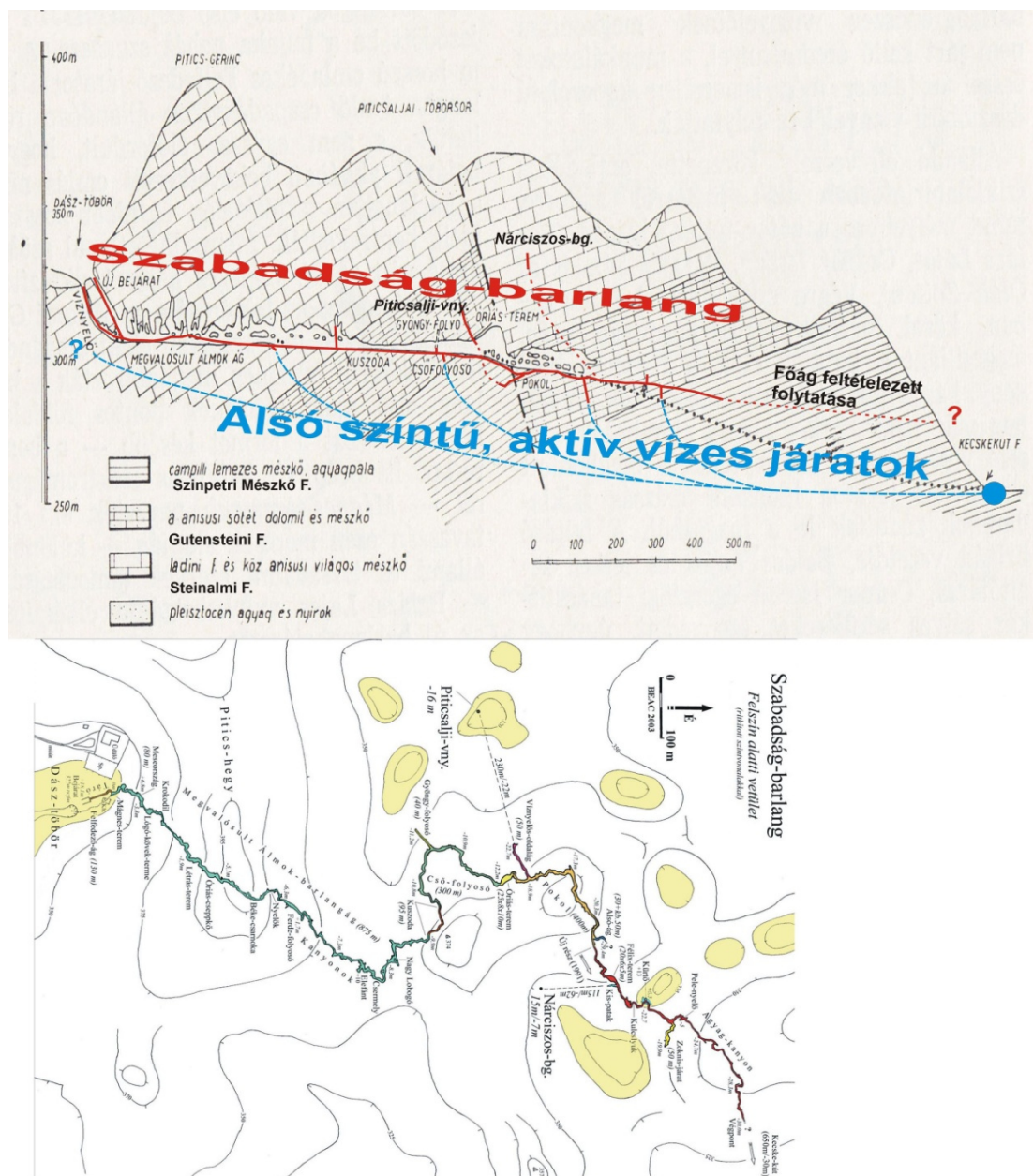
22. ábra A Szabadság-barlang térképe, hosszelvénnyé és poligonvonala a feltételezett ismeretlen járatokkal ( BALÁZS 1962 és a Tájvédelmi, Barlangvédelmi és Ökoturisztikai Osztály térképe alapján kiegészítve)
