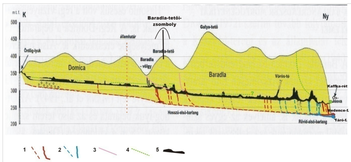
20. ábra A Baradla-rendszer kiterített hosszszelvénye (Gaál L.(2014) alapján kiegészítve szerkesztette: Sásdi L.)
