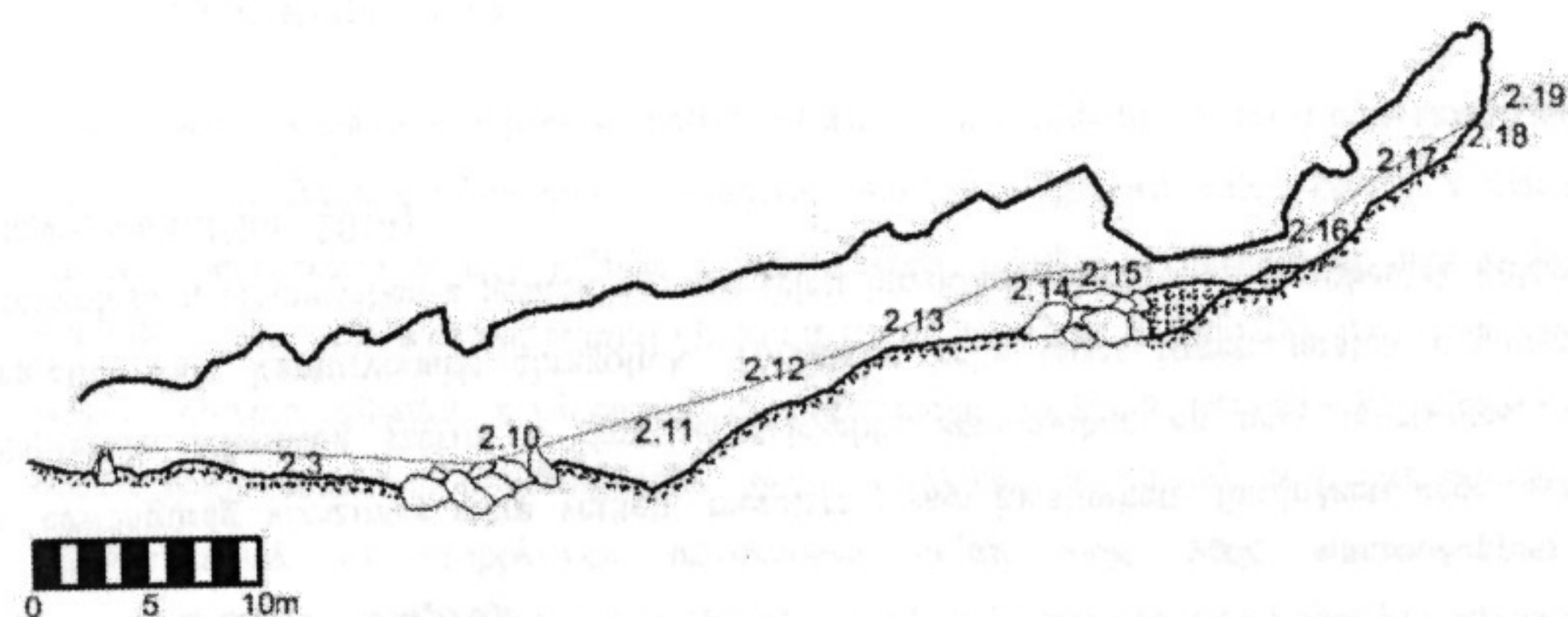
4. ábra Óriások-útja – oldalnézet
