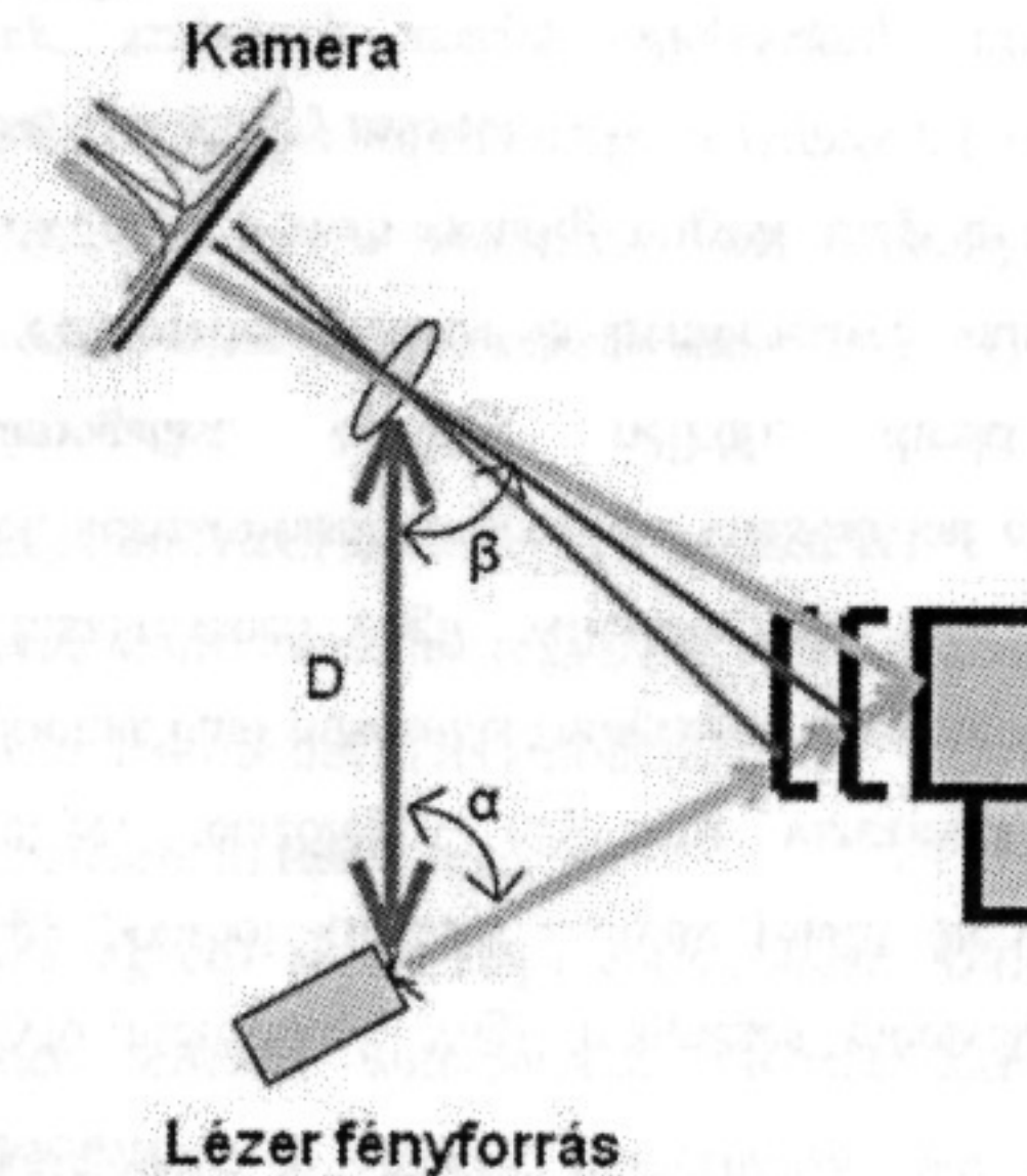
6. ábra Háromszögelés elvén alapuló szkennер (Tarsoly, 2010)
