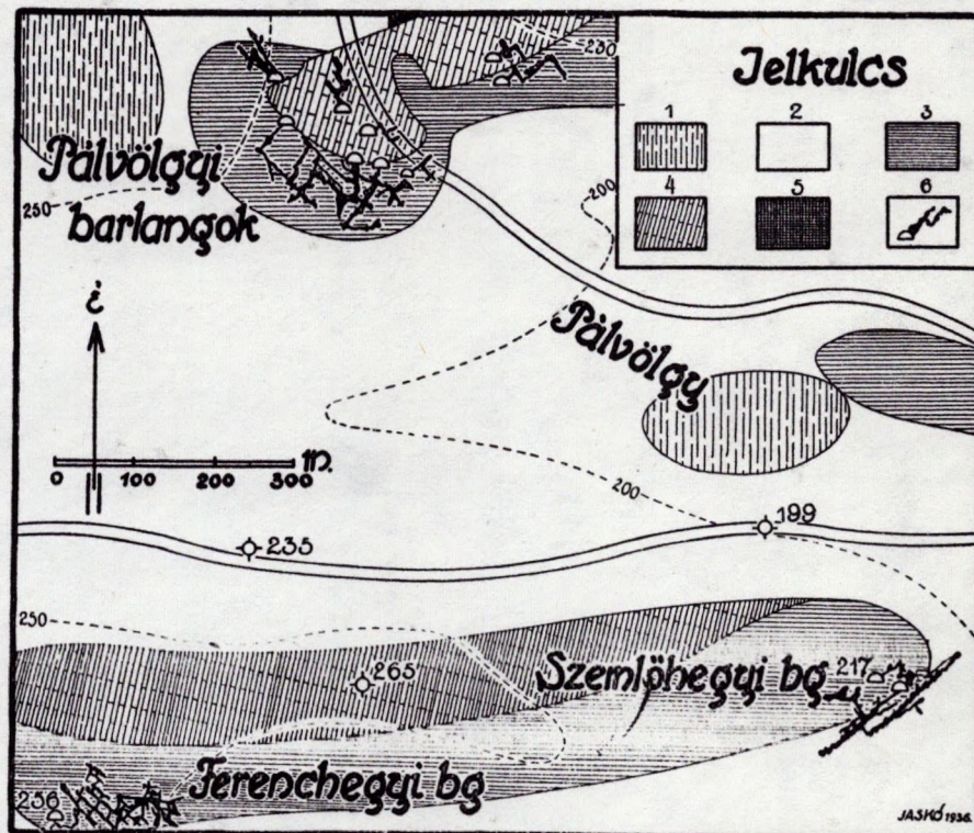
1. kép. A Pálvölgy—Rózsadombi barlangvidék földtani térképe. 1 = lösz (pleisztocén), 2 = budai márga (oligocén), 3 = bryozoás márga (eocén), 4 = nummulinás-orbitoidás mészkő (eocén), 5 = f. triász raibli mészkő, 6 = barlangok (a félkör a bejárat nyílását, a feketén kihúzott rész a járatok alaprajzát mutatja.)
