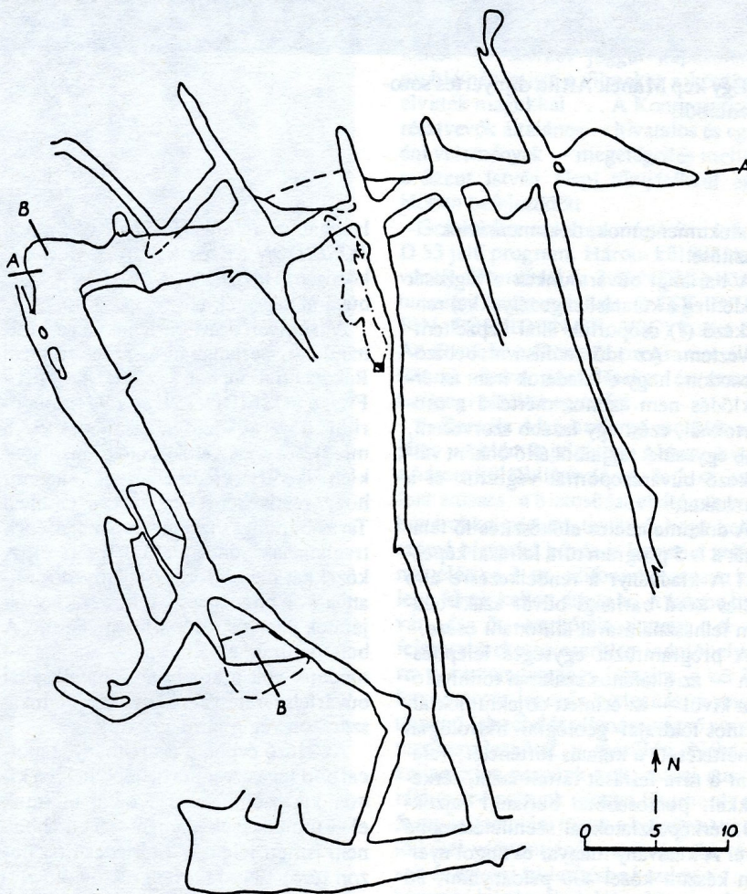
Molnár János-barlang alaprajz
