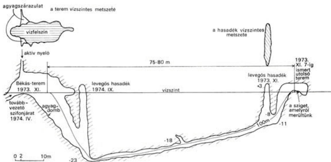
A Csarnóházi-forrásbarlang 1973. XI. 7–10-én feltárt szifonjának vázlatos képe. A későbbi merülések alapján korrigált változat (Mozsáry G.)
