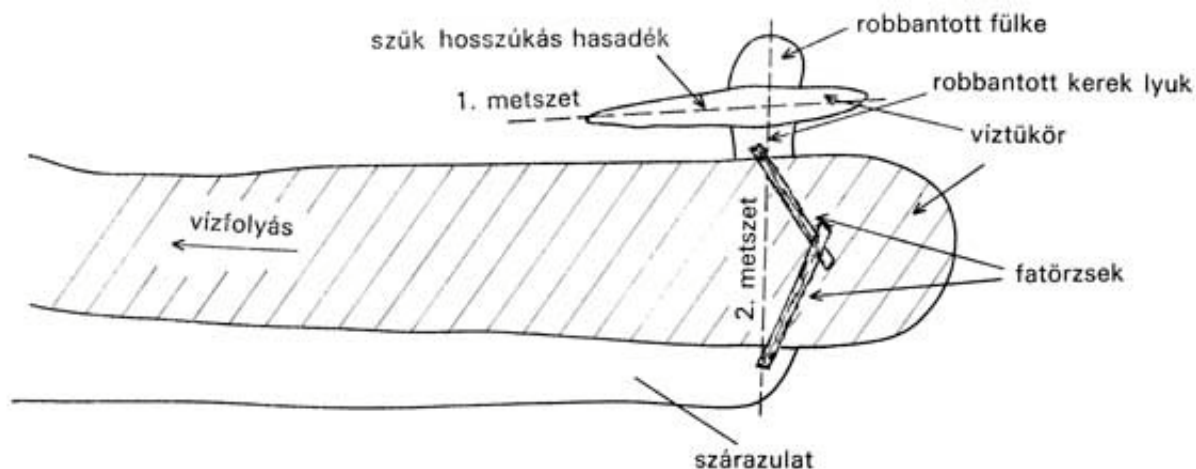
A Kossuth-barlang szifon körüli részének vázlatos rajza
