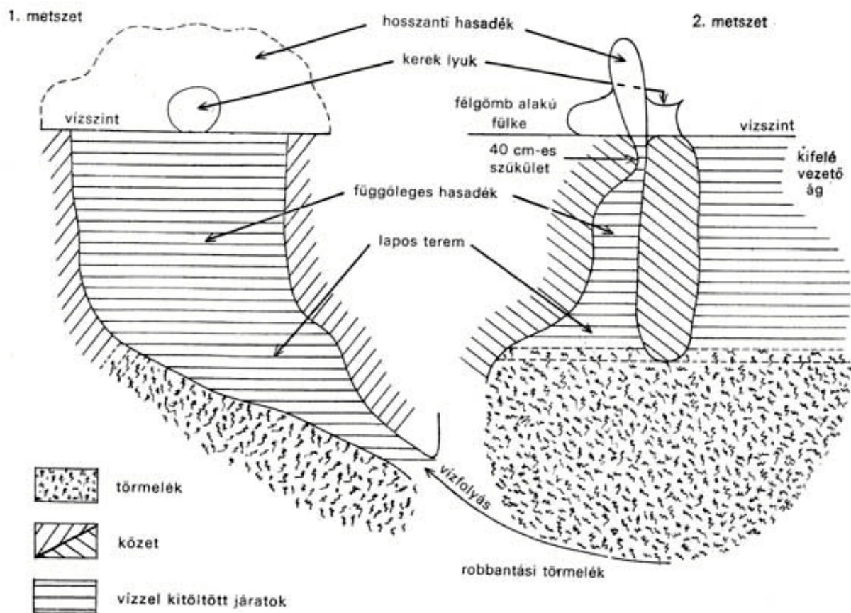
A szifon függőleges metszete
