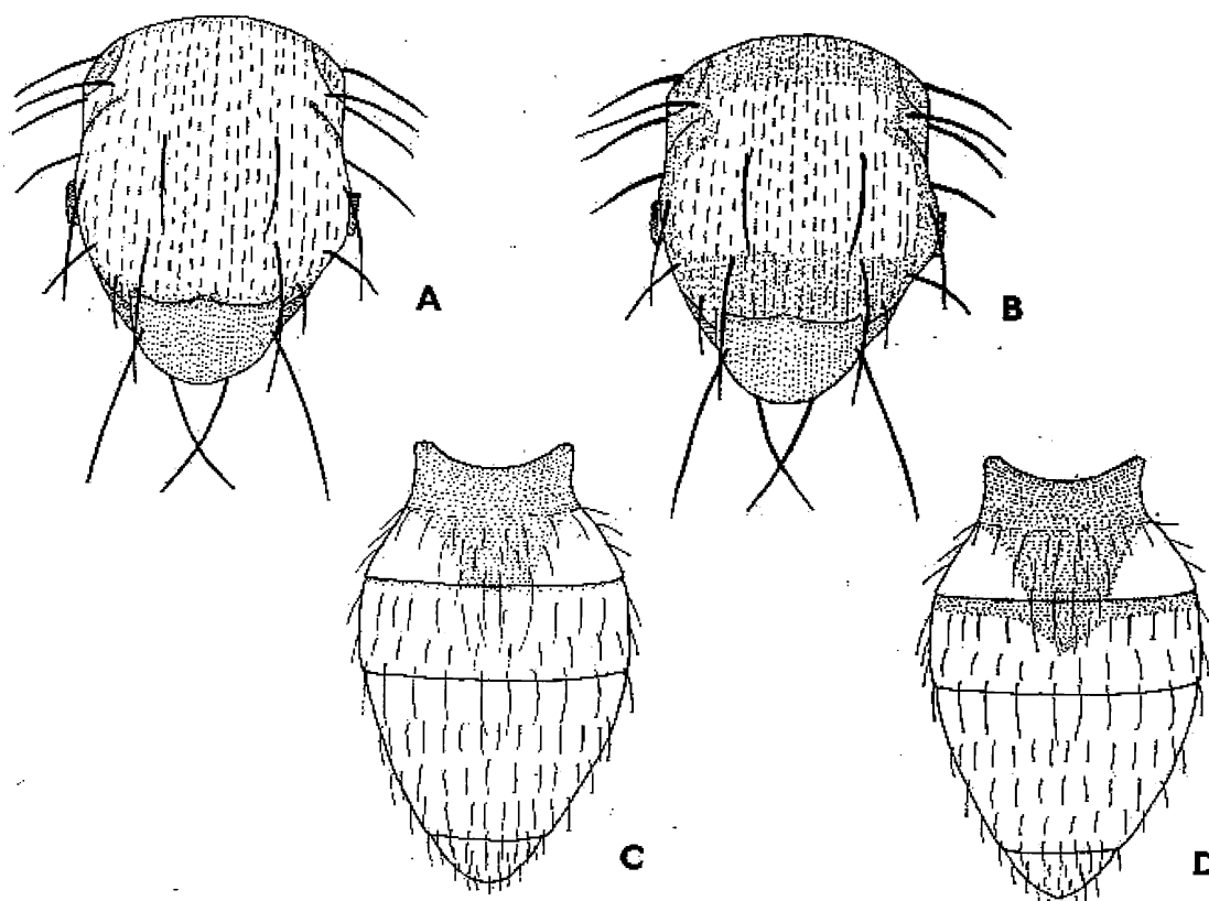
63. ábra. A: Camilla glabrata COLL. és B: C. nigrifrons COLL. tóra — C: C. glabrata COLL. és D: C. nigrifrons COLL. potroha (Eredeti)
