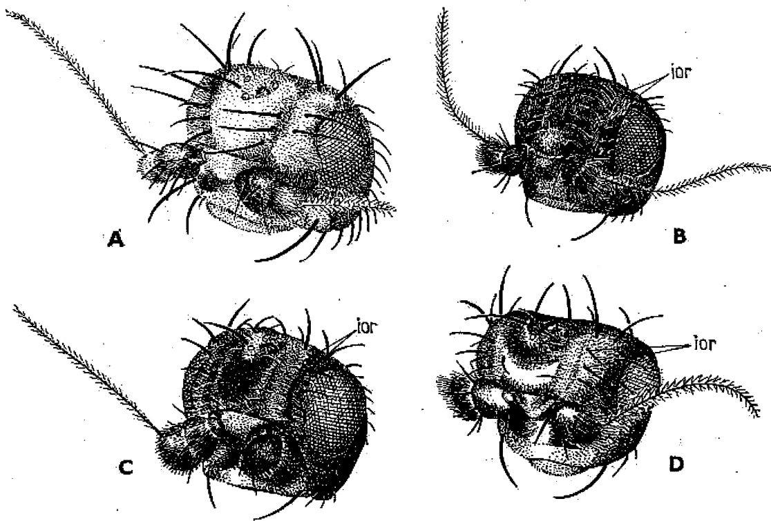
21. ábra. A: Thoracochaeta zosteræ HALID., B: Elachisoma pilosa DUDA, C: Halidayina spinipennis HALID., és D: Trachypella leucoptera HALID. feje (ior = belső orbitalis sörtek) (Eredeti)
